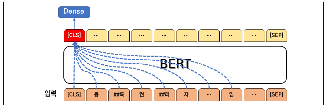
<그림4 버트 컨텍스트 벡터인 [CLS] 토큰을 활용한 특허상담 텍스트 데이터 임베딩 예시>
