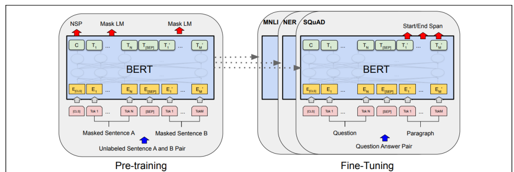
<그림2 버트(BERT)의 사전 훈련 및 파인튜닝> 10)
