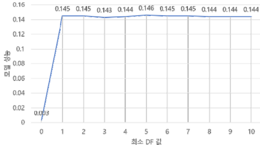
<그림 5 Logistic Regression 모델의 최소 DF 값 설정 실험>
