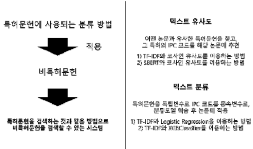
&lt;그림 2 연구 절차&gt;
