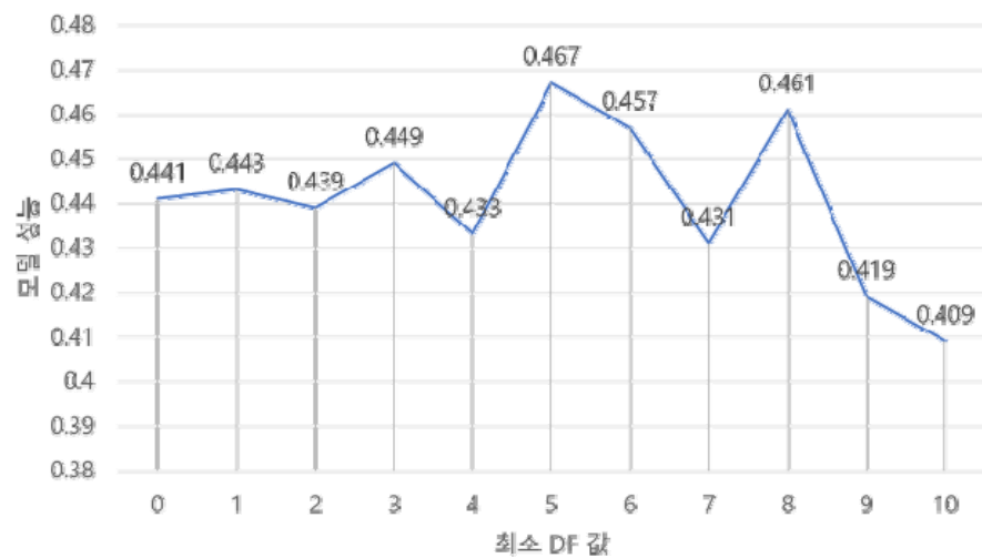
<그림 6 XGBClassifier 모델의 최소 DF 값 설정 실험>
