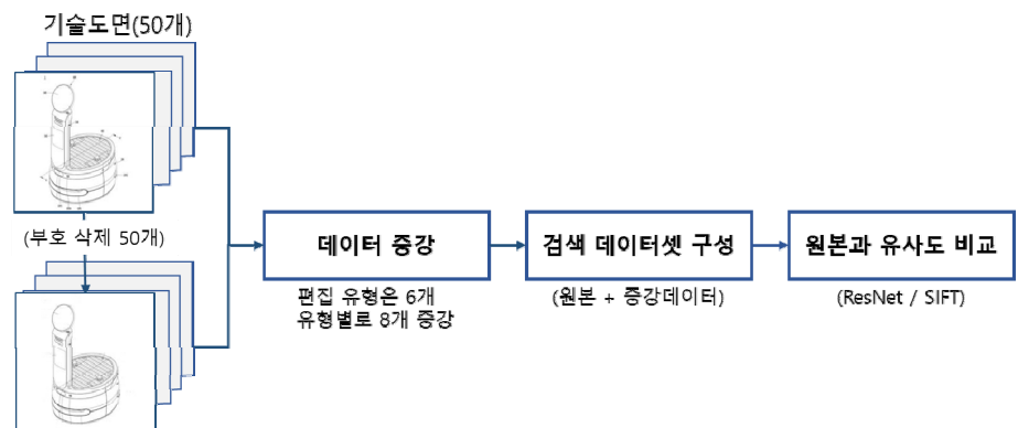
<그림7 증강데이터를 이용한 유사도 비교 프로세스>
