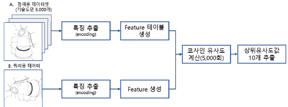
&lt;그림5 ResNet을 이용한 유사도 비교 프로세스&gt;
