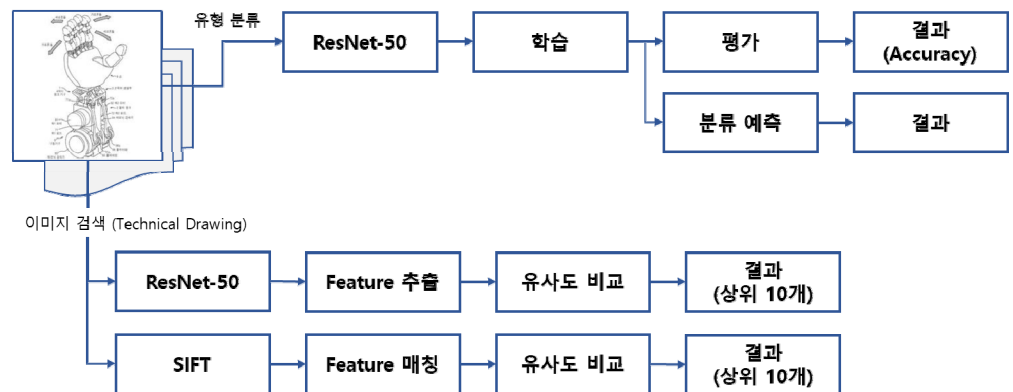
<그림3 특허도면의 유형분류 및 검색 실험 프레임워크>
